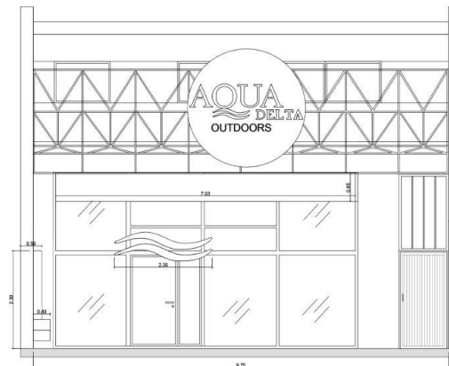
FACHADA
