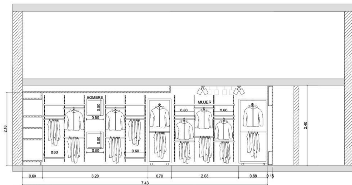
CORTE C-C
