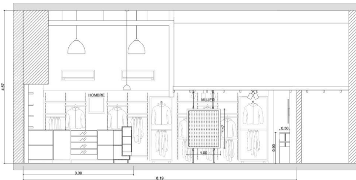
CORTE D-D
